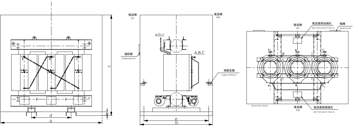
图2 SCB10 (11, 12) - 630~2500 kVA 下进下出 Fig.2 SCB10 (11, 12) - 630~2500 kVA bottm in-bottm out
