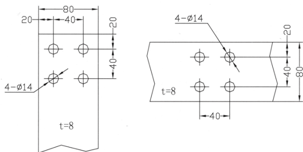
图 Fig.5(o, a, b, c)
