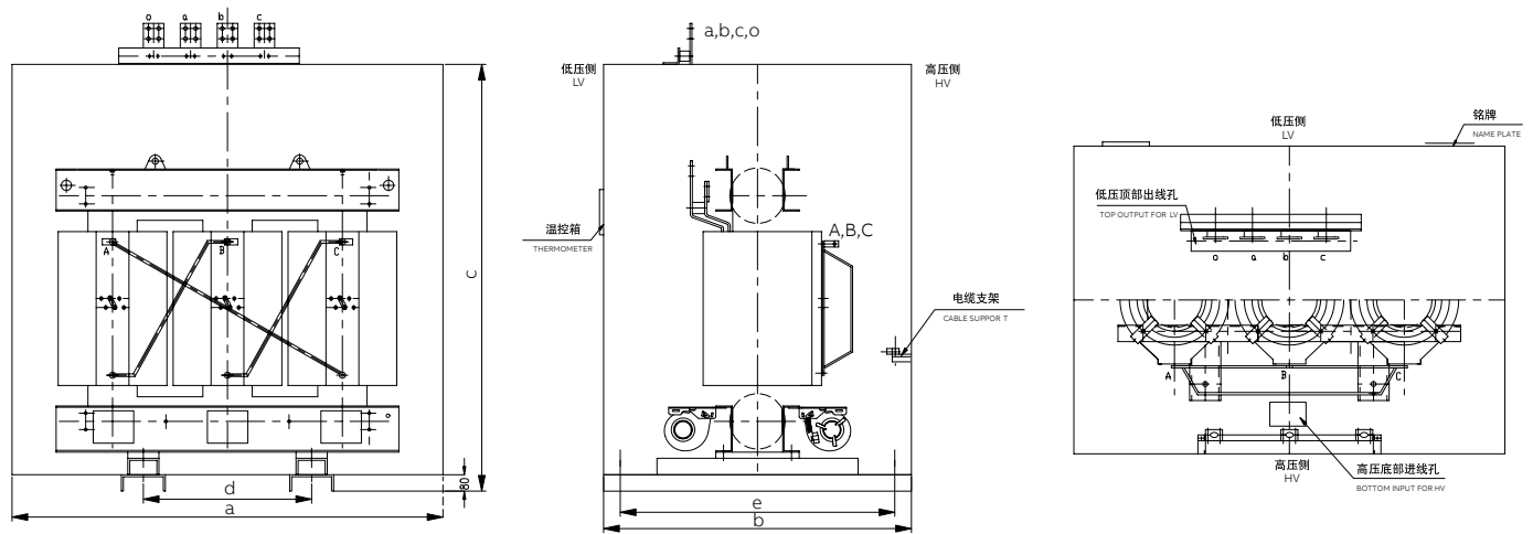
图3 SCB10 (11, 12) - 630~2500 kVA 下进上出
